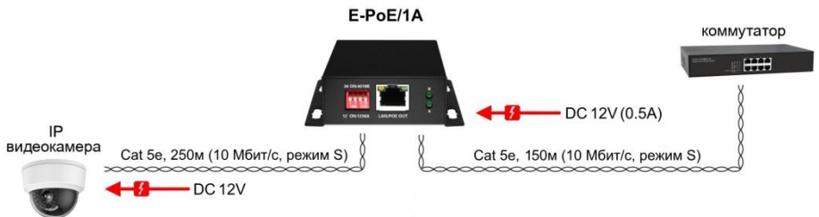
Рис.5 Схема подключения удлинителя E-PoE/1A в режиме удлинения Ethernet
