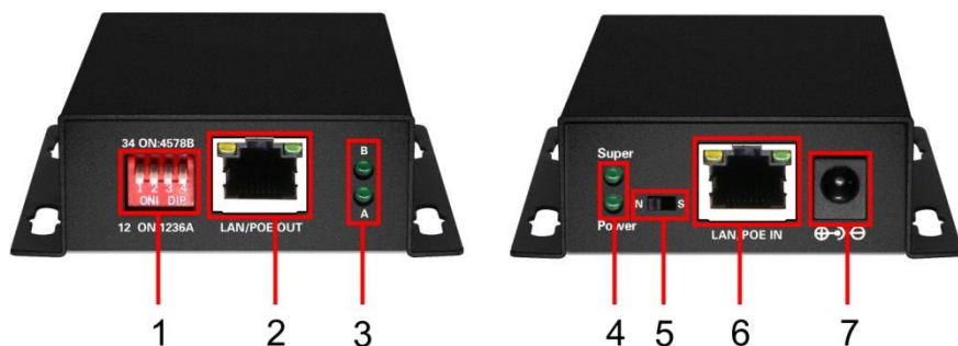
Рис. 2 Панели подключения удлинителя E-PoE/1A
