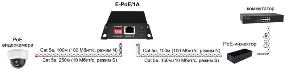
Рис.3 Типовая схема подключения удлинителя E-PoE/1A в режиме питания от PoE инжектора
