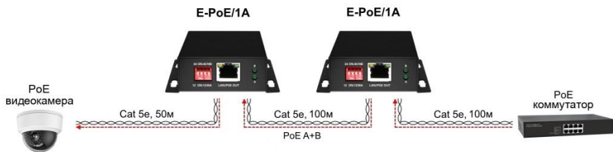
Рис.6 Схема подключения удлинителя E-PoE/1A в каскадном режиме
