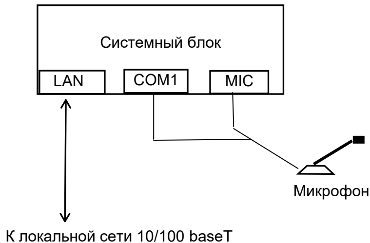
Рис.6. Схема подключения пульта СДК-330S1
